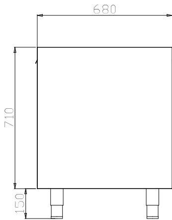
Zij aanzicht
